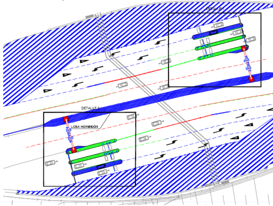
PÓRTICO DE 14M DE LUZ Y 6 m DE GÁLIBO
