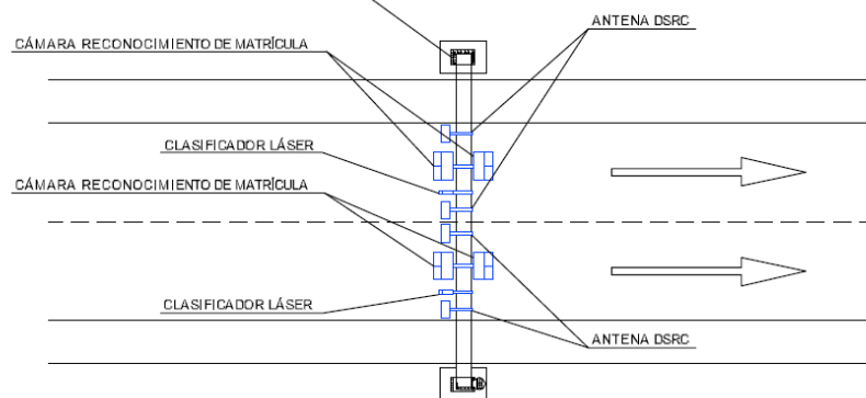
PÓRTICO DE 14M DE LUZ Y 6 m DE GÁLIBO
