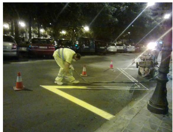
Ejecución de marcas viales
