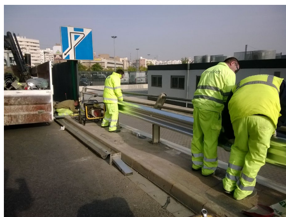
Montaje de barrera de contención
