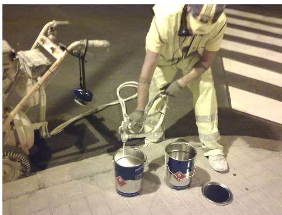
Control de calidad de la pintura empleada para la ejecución de marcas viales
